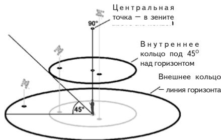
Изображение небосвода
